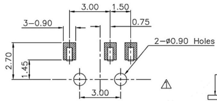
PCB Layout(Pattern TOP)
